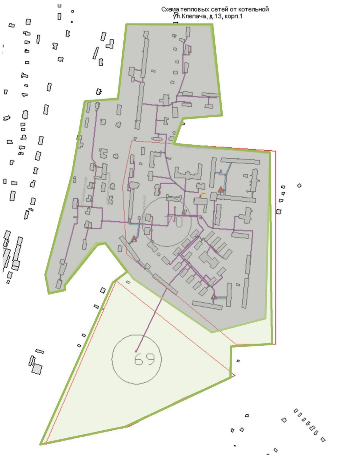
Рисунок 2.3. Предлагаемая зона деятельности №28 (существующее и перспективное состояние)
